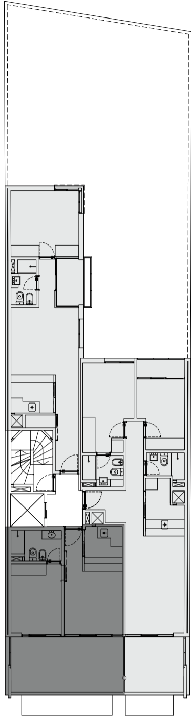
PLANTA PENTHOUSE UNIDAD 01 ESC. 1.200
