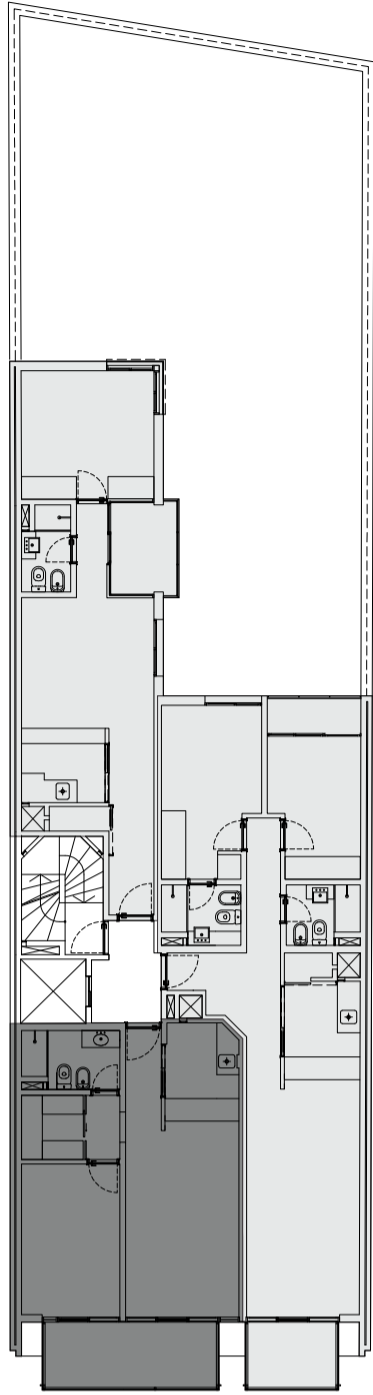
PLANTA TIPO UNIDAD 01 ESC. 1.200
